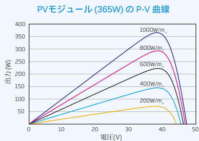
PVモジュール (365W) の P-V 曲線
